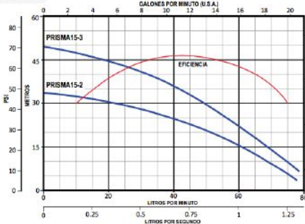
CURVAS DE RENDIMIENTO PRISMA 15
