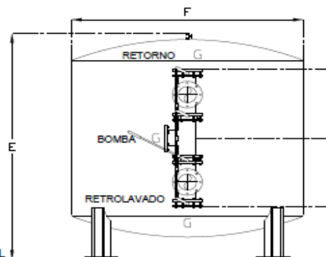
SECCION LATERAL
