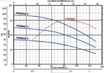
CURVAS DE RENDIMIENTO PRISMA 25
