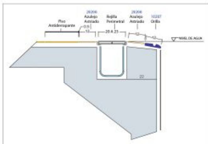
Esquema de instalación (medidas en cm)
